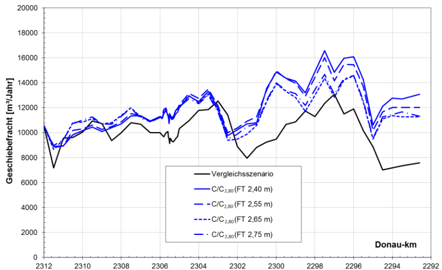
Abb. 5 Berechneter mittlerer Geschiebefrachtlängsschnitt in \text{m}^3/\text{Jahr} (sogenanntes Transportdiagramm) für die Variante C/C_{2,80} sowie den Bestand (Vergleichsszenario) für die Ganglinie 2001 bis 2003.
