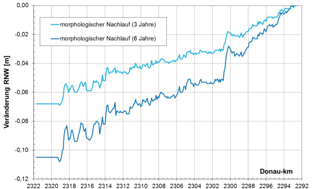
Abb. 4 Veränderung des RNW Wasserspiegels aufgrund des morphologischen Nachlaufes in 3 bzw. 6 Jahren bei Variante C/C 2,80 .
