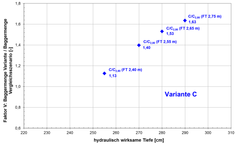
Abb. 6 Verhältnis der Baggermengen auf dem Abschnitt Fkm 2310 – 2296 für die Variante C/C 2,80 gegenüber dem Vergleichsszenario.
