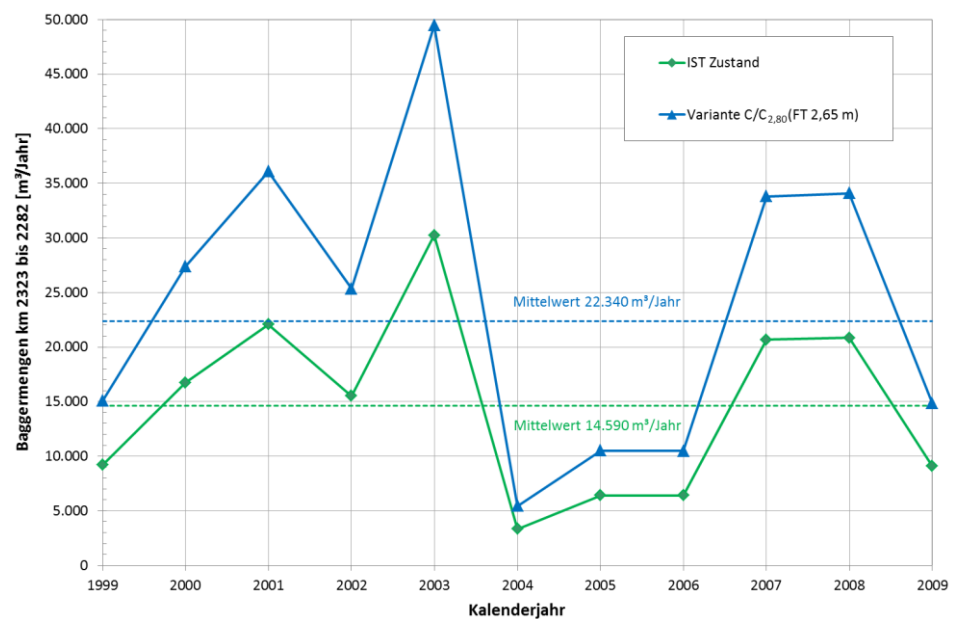
Abb. 7 Baggermengen im IST- und im Planungszustand für Variante C/C 2,80 .
