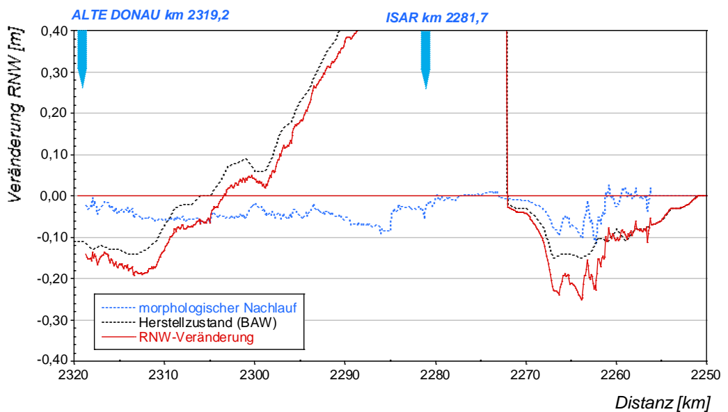
Abb. 3 Auswirkungen der Variante C/C 2,80 auf den RNW-Wasserspiegel (rote Linie) 7 unter Berücksichtigung der Regelung (schwarze Linie) und des morphologischen Nachlaufs (blaue Linie).
