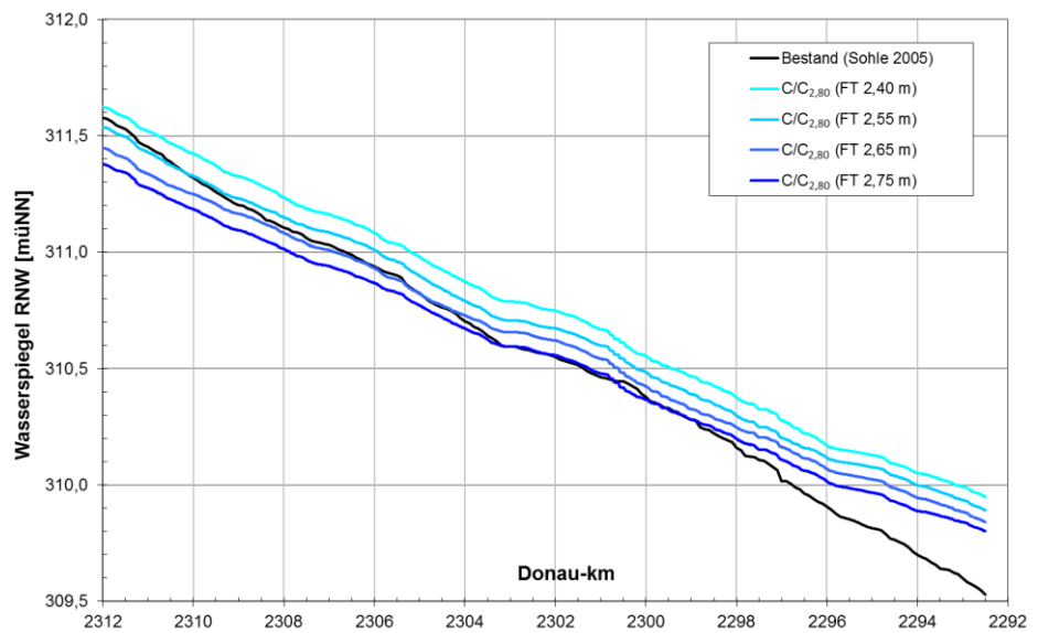
Abb. 3: Vergleich des heutigen (neu berechnet auf Basis Sohle 2005) mit den zukünftigen Bezugshorizonten RNW bei einem Abfluss von 211 \text{ m}^3/\text{s} .
