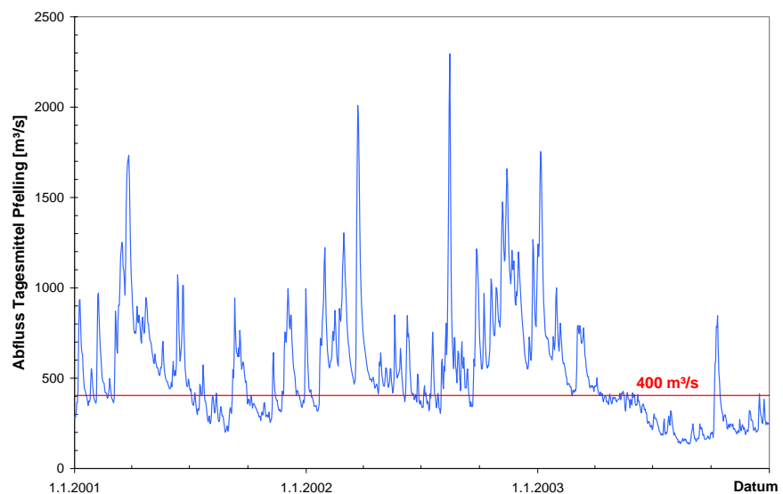
Abb. 4: Abflussganglinie am Pegel Pfulling in der Periode 2001 bis 2003.
